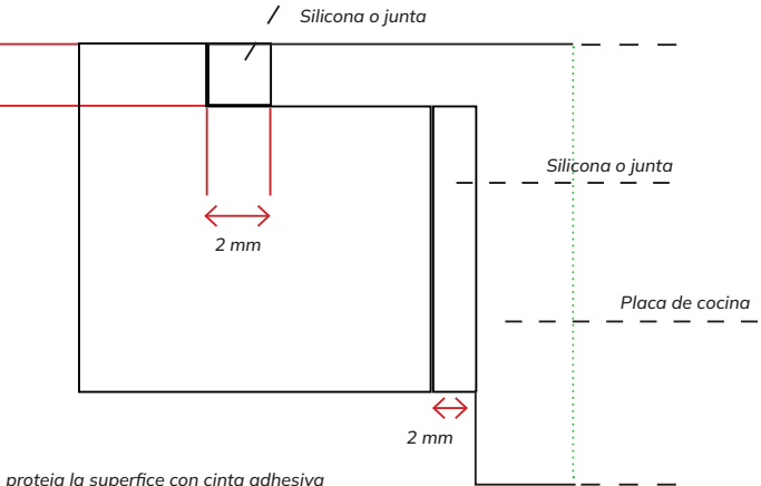
Placa de cocina a ras de la encimera
